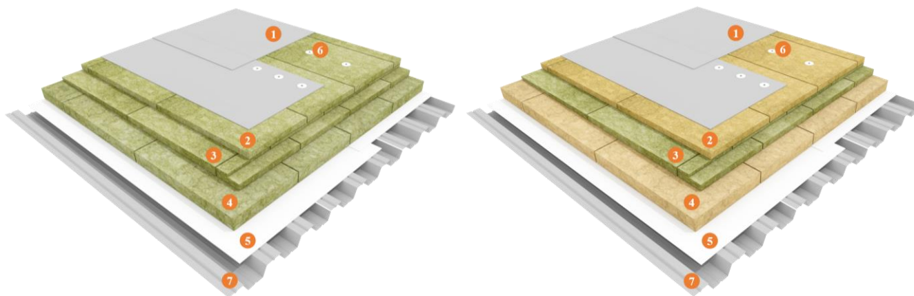
Рис. 1. Конструкция кровельной системы по профилированному основанию с использованием минеральной изоляции и ПВХ-мембраны
