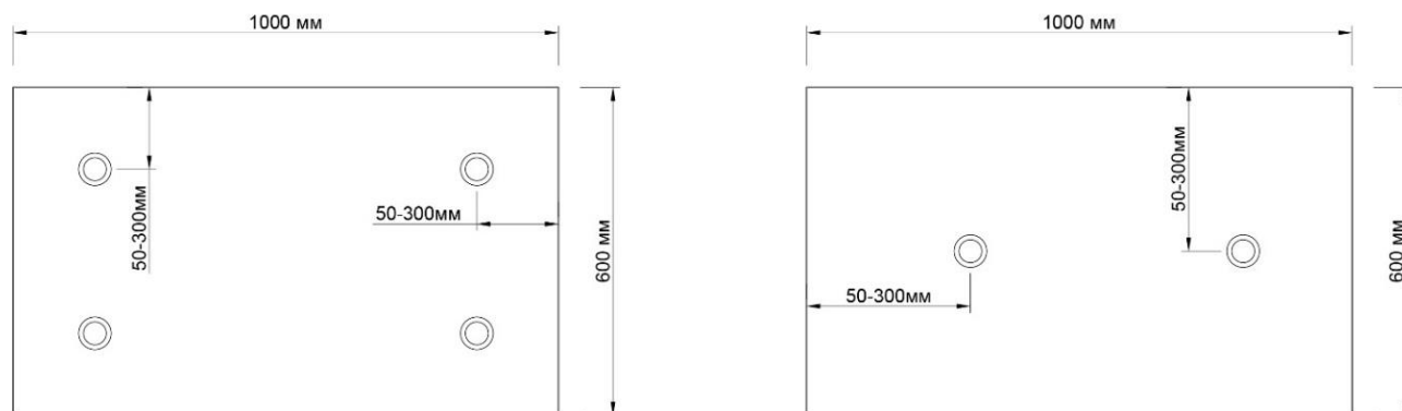
Рис.11. Схема крепления теплоизоляционных плит из минеральной ваты
