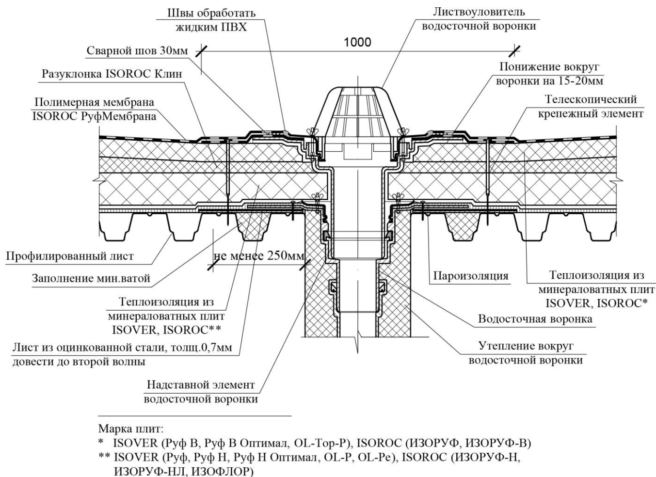
Рис. 20 Водоприемная воронка
