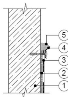
Рис. 26. Закрепление края кровельного ковра металлической краевой рейкой. Вариант 2.
