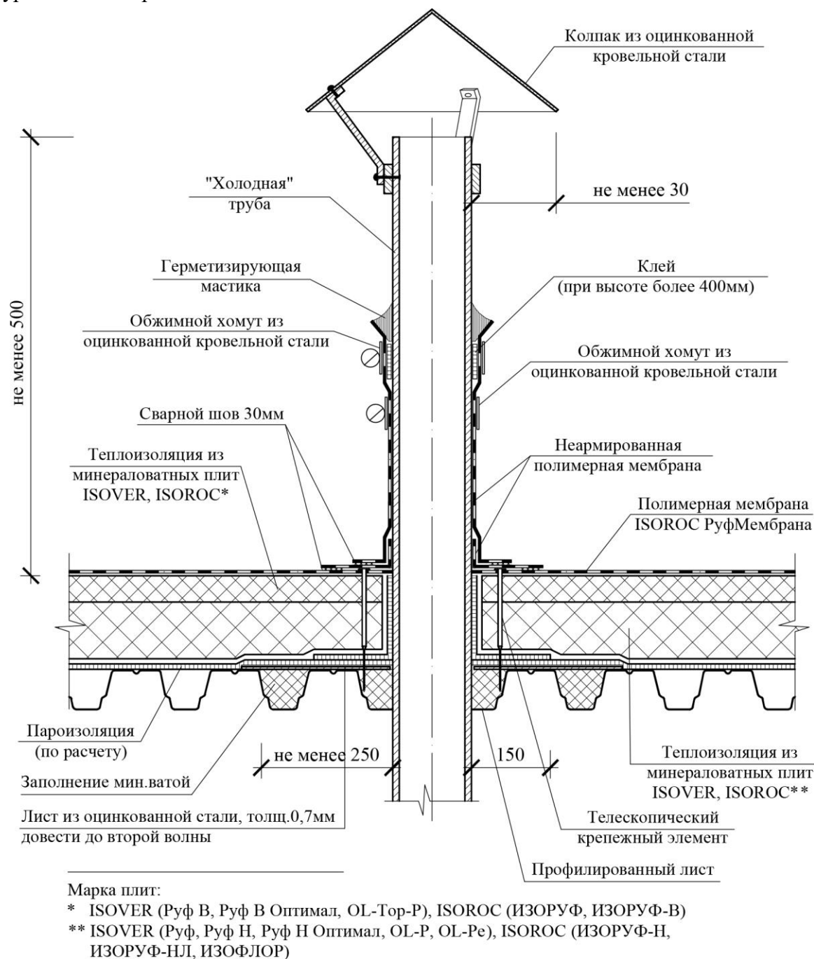
Рис.35. Примыкание кровли к «холодной» трубе
