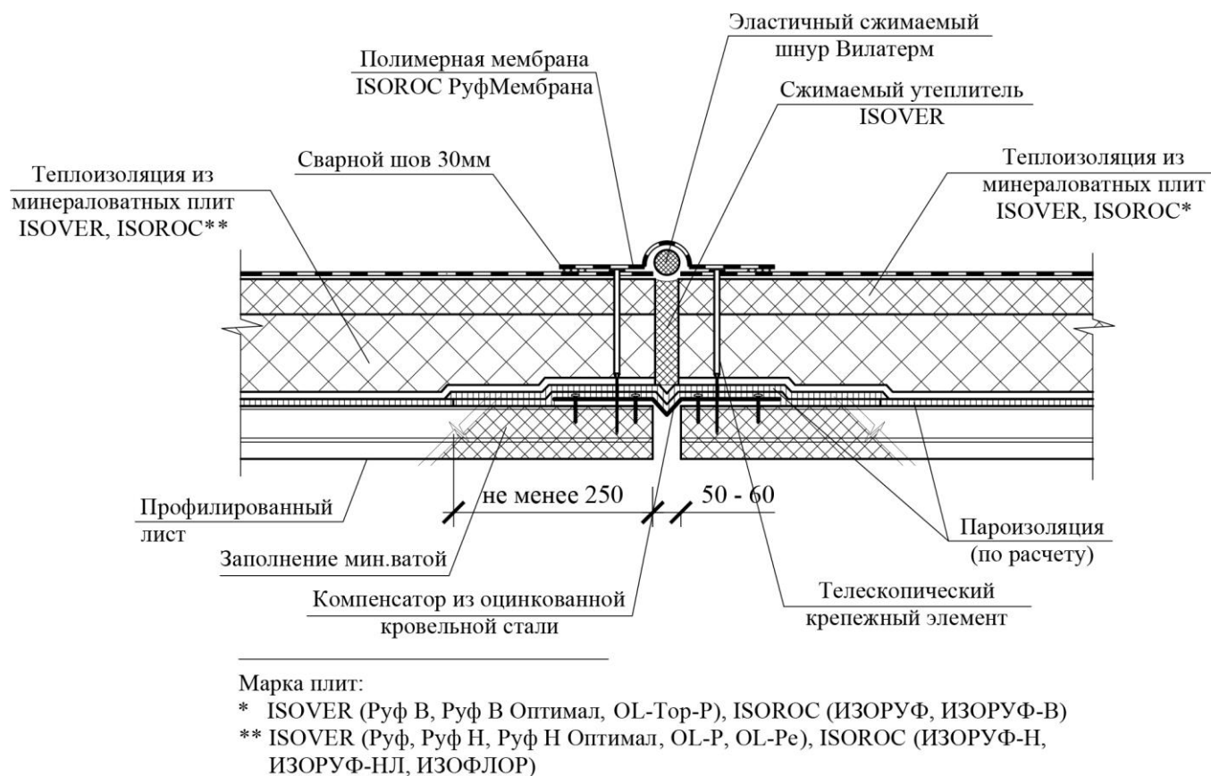
Рис. 36. Деформационный шов. Вариант 1
