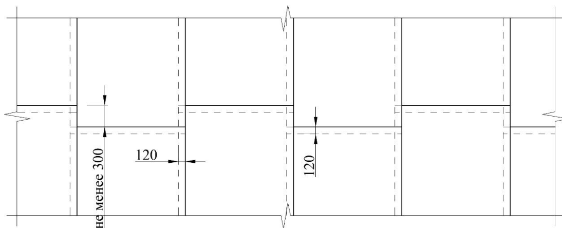
Рис.14. Вариант раскладки рулонов полимерной гидроизоляционной мембраны
