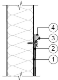
Рис. 21 Закрепление края кровельного ковра металлической краевой рейкой. Вариант 1. 1 – гладкая поверхность; 2 – кровельный материал; 3 – краевая рейка; 4 – герметик полиуретановый.
