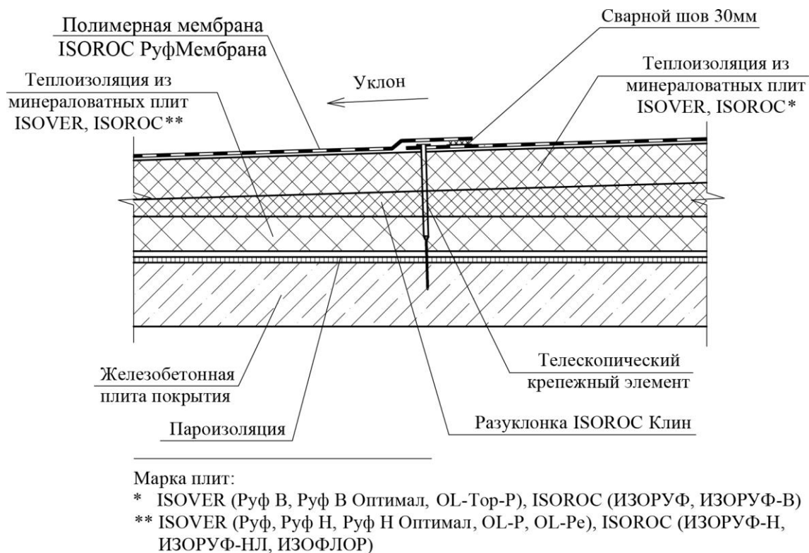
Рис. 15 Устройство гидроизоляционного кровельного ковра из ПВХ-покрытия. «Встречный» шов»
