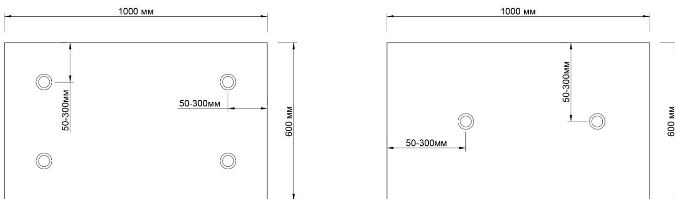
Рис.11. Схема крепления теплоизоляционных плит из минеральной ваты.
