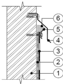
Рис. 27. Примыкание кровли к стене с механическим креплением края кровельного ковра
