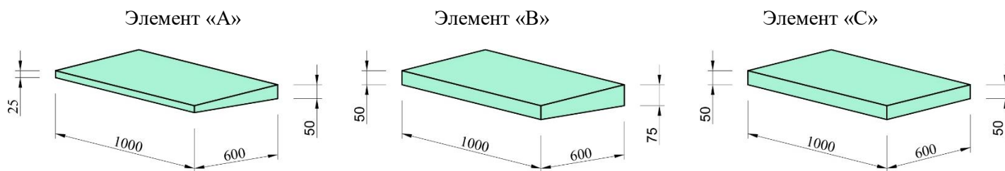
Рис.6. Набор плит ISOROC Клин «А», «В» 4,2% и добор толщиной 50мм – «С»
