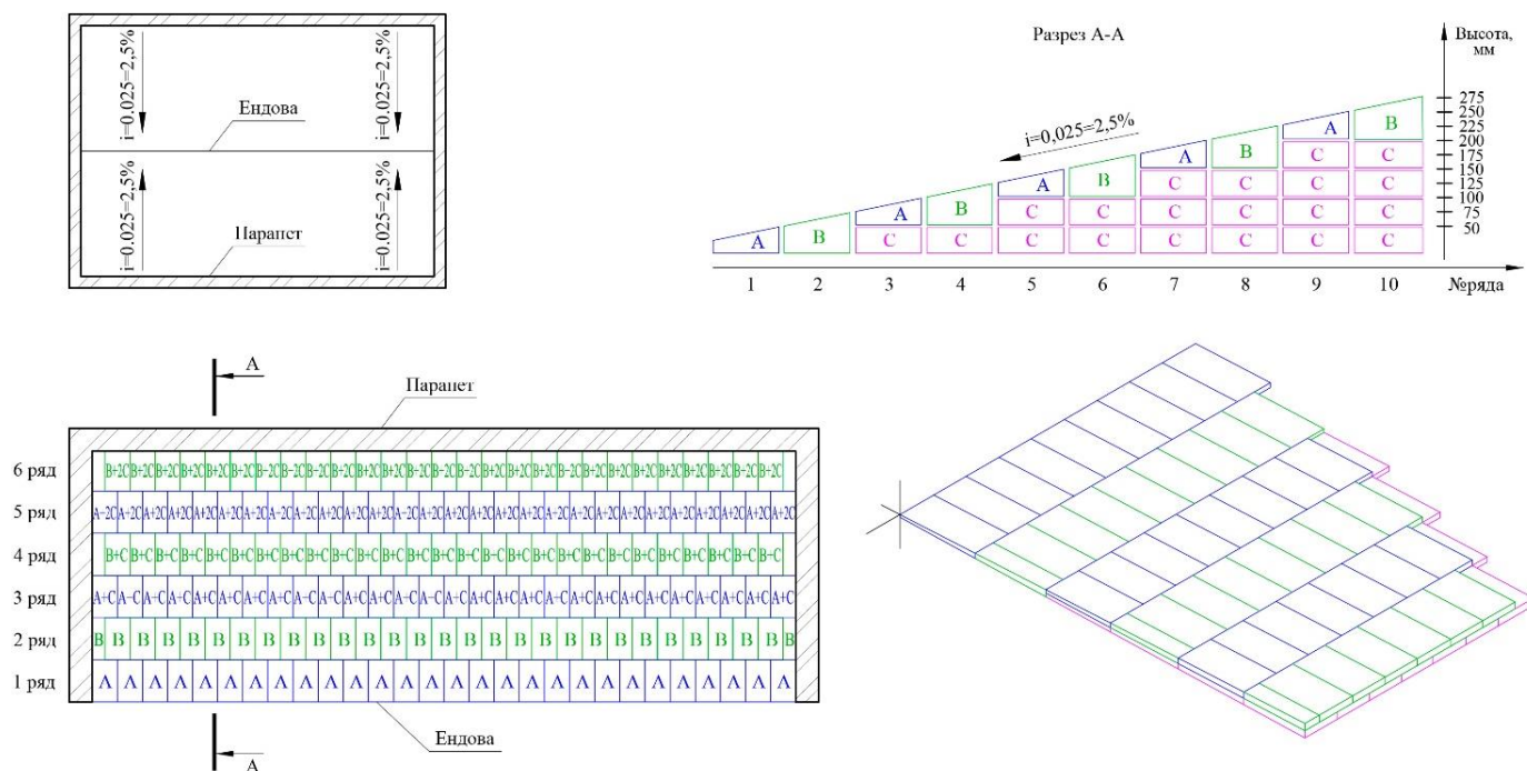
Рис.5. Пример выполнения основного уклона из плит ISOROC Клин 2,5%
