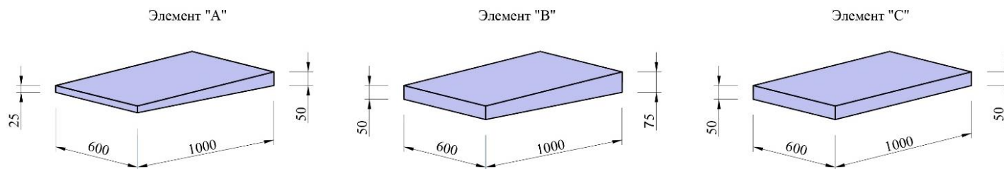
Рис.4. Набор плит для основного уклона ISOROC Кли́н; 2,5%
