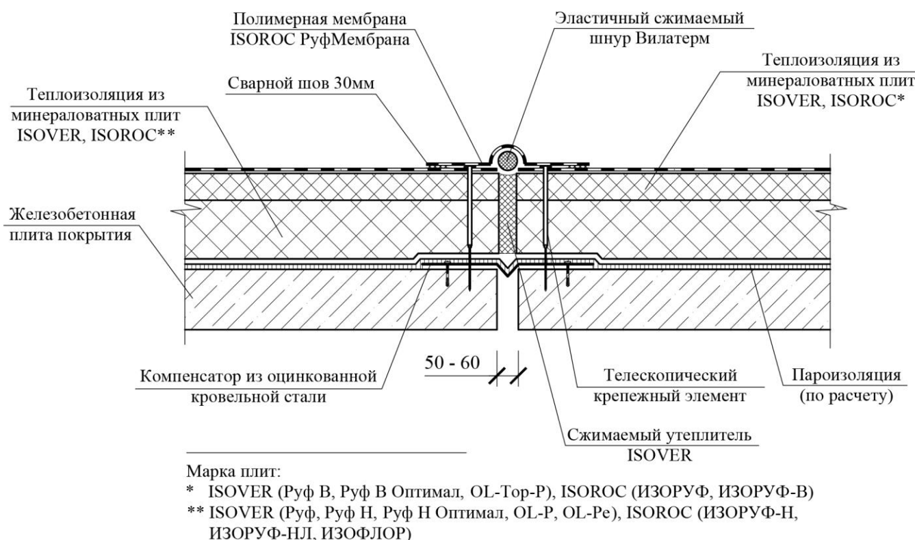
Рис. 33. Деформационный шов Вариант 1
