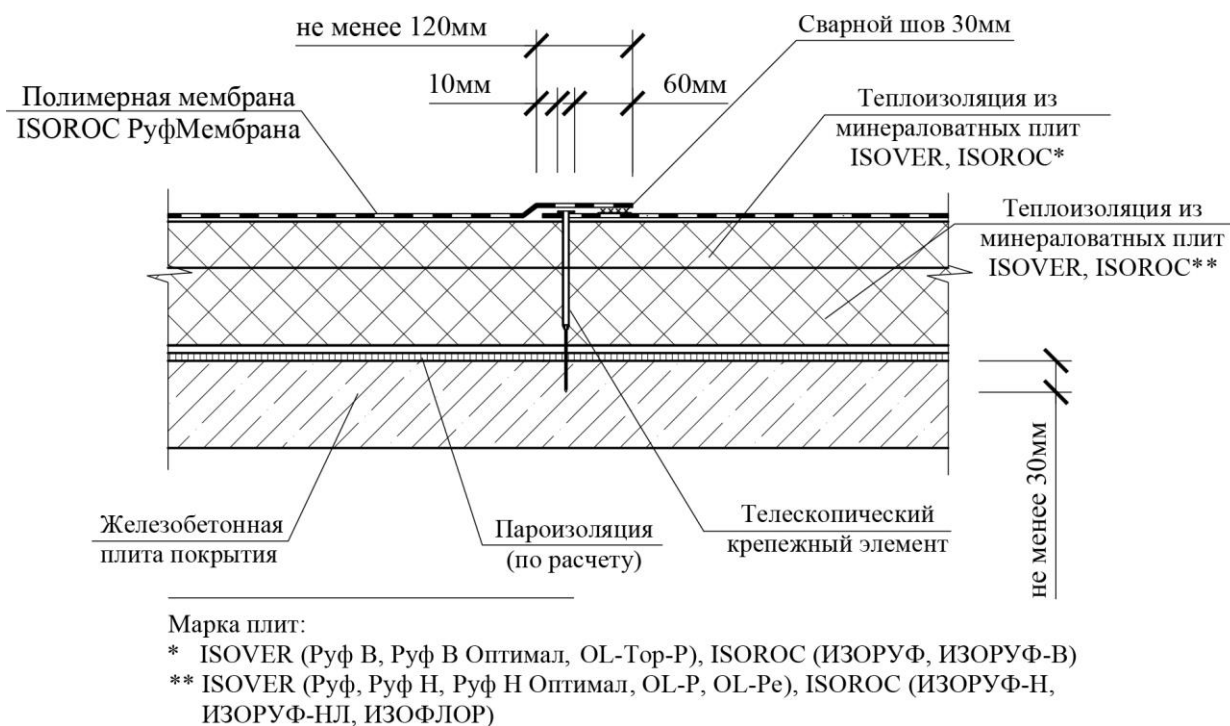
Рис. 13. Устройство гидроизоляционного кровельного ковра из ПВХ-покрытия
