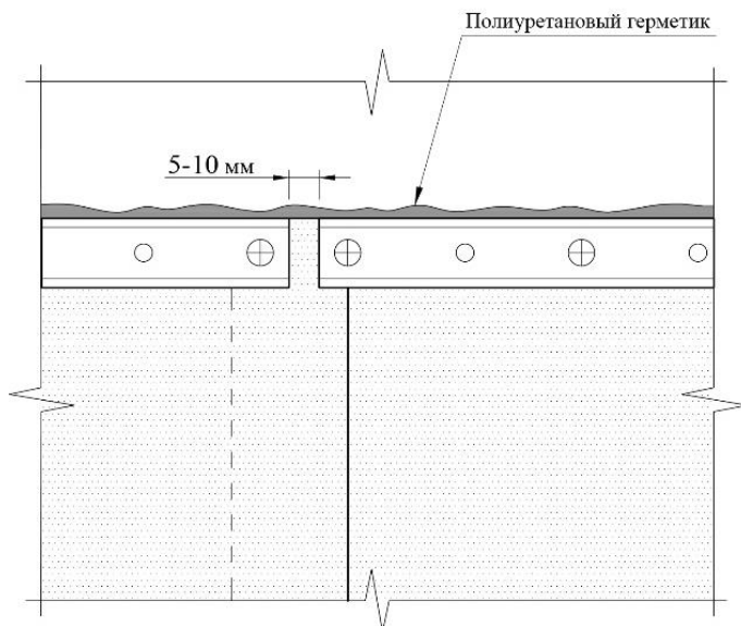
Рис. 28. Зазор между краями соседних реек
