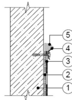
Рис. 22 Закрепление края кровельного ковра металлической краевой рейкой. Вариант 2. 1 – шероховатая поверхность; 2 – геотекстиль; 3 – кровельный материал на вертикальной поверхности; 4 – краевая рейка; 5 – герметик полиуретановый
