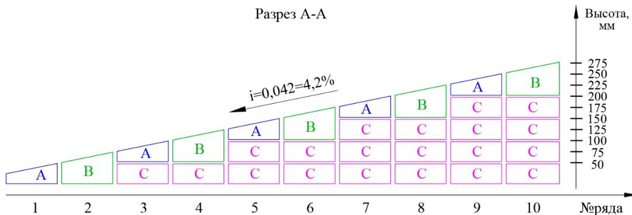
Рис.8. Схема послойной укладки плит ISOROC Клин 4,2% при создании разуклонки между воронками в ендове.
