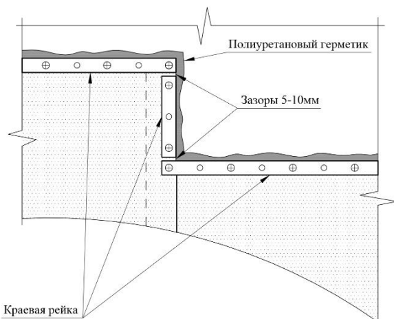
Рис. 30. Обрамление края кровельного ковра краевой рейкой
