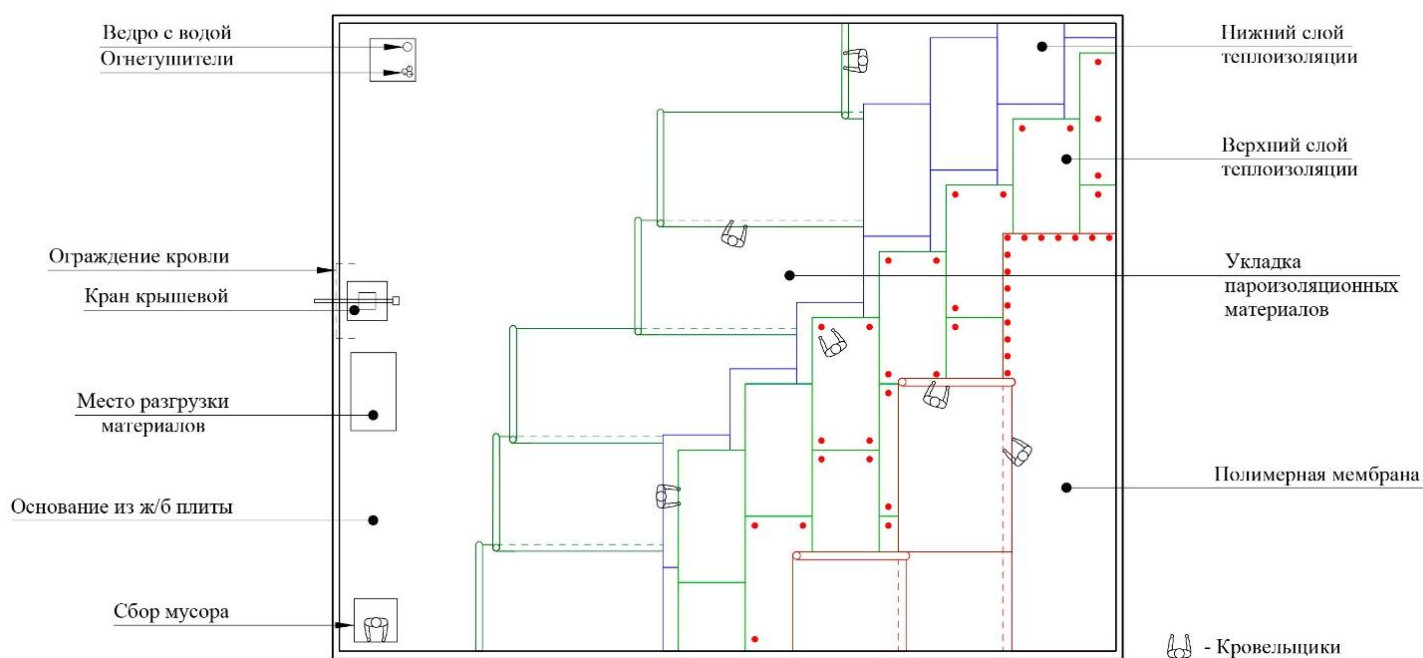
Рис. 2. Схема организации рабочего места
